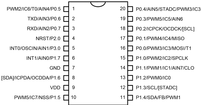
图4-1. XM003Q TSSOP-20 封装管脚配置
