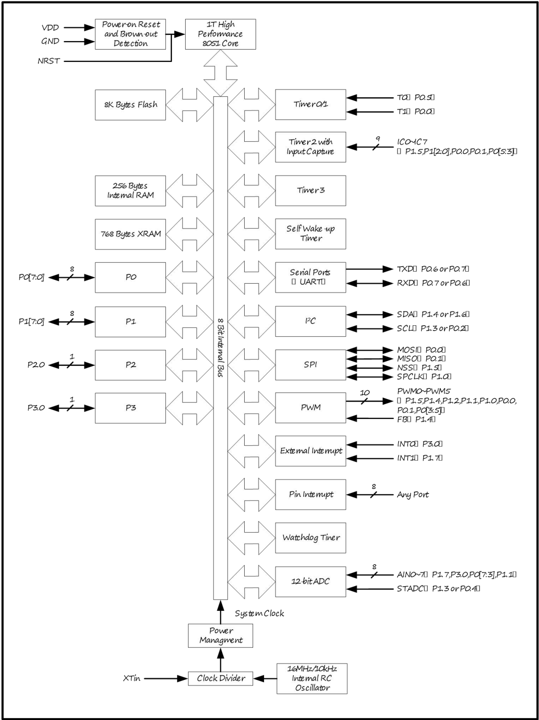
图 3 - 1. 功能方块图
