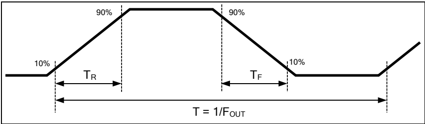
图30-1. I/O AC 电气特性定义图
